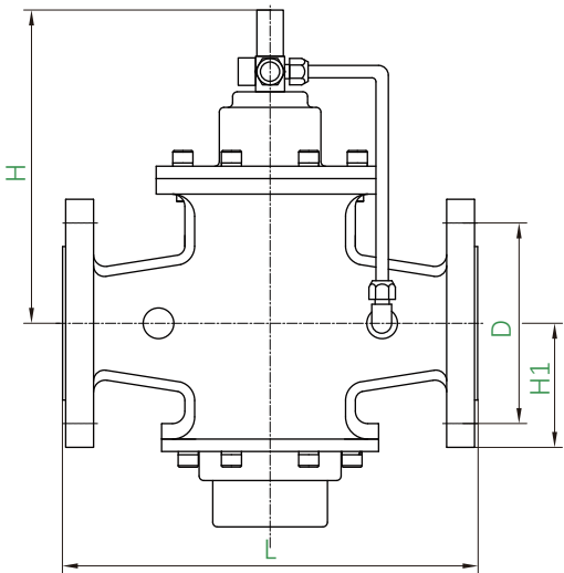
DN300- DN500
