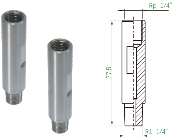
延长杆
